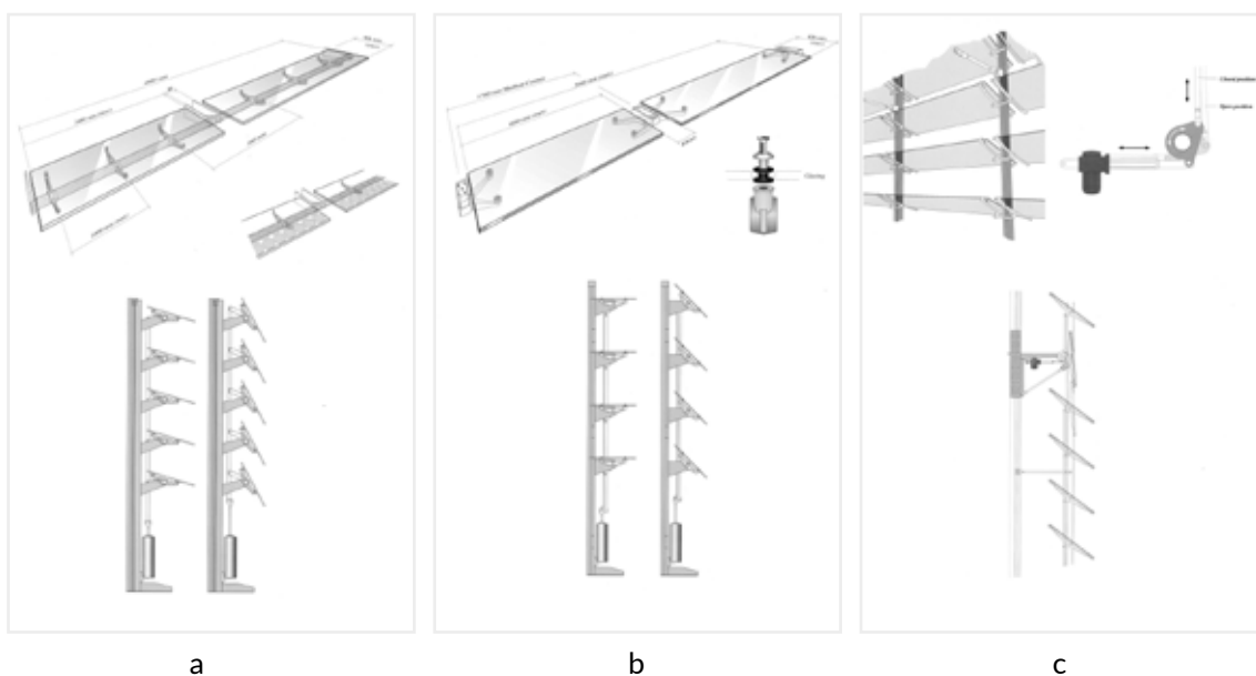
16. Installazione esterna mobile: dispositivi frangisole orientabili a pale.
