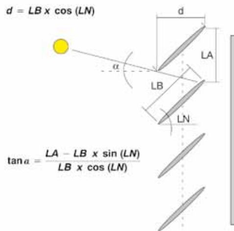
34. Calibrazione esecutiva e regolazione funzionale. Le schermature solari sono applicate secondo l'incidenza della radiazione solare diretta, le condizioni luminose durante l'inverno, la quota proiettiva orizzontale delle lamelle (d), la di-stanza tra le lamelle (LA), l'ampiezza delle lamelle (LB), l'angolazione delle lamelle (LN) e l'angolo critico di incidenza solare ( \alpha ).
