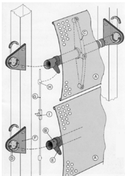
14. Installazione esterna mobile: dispositivi frangisole orientabili a pale.
