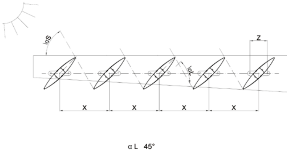
36. Calibrazione esecutiva e regolazione funzionale.
