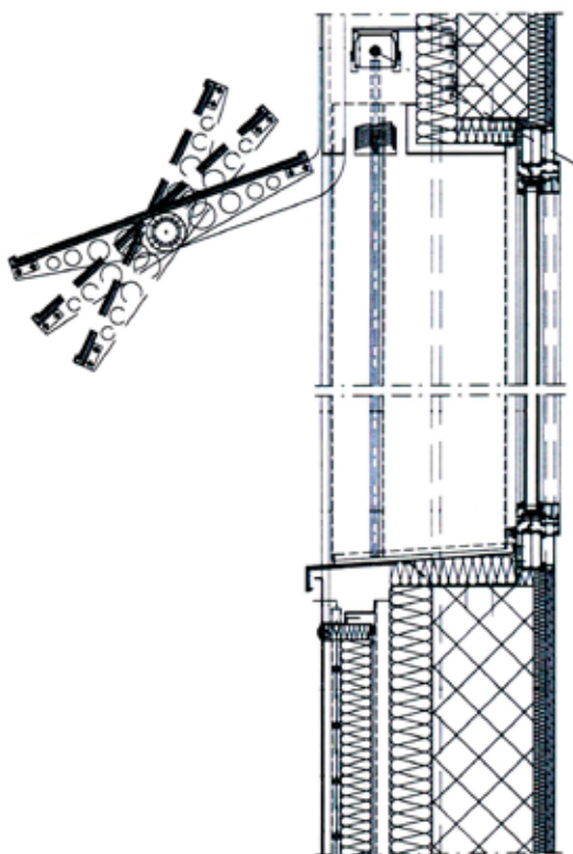
31. Combinazione con moduli fotovoltaici.
