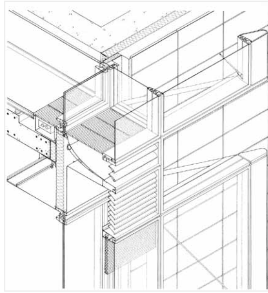
30. Installazione integrata (facciata).
