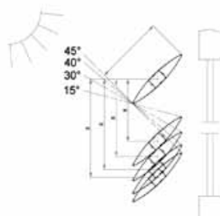
35. Calibrazione esecutiva e regolazione funzionale. La costruzione considera l'angolazione delle lamelle ( \alpha L ) rispetto all'asse verticale e la distanza di esecuzione (X) tra gli assi delle lamelle in funzione dell'angolo critico di incidenza solare.
