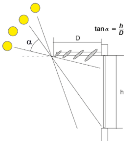
33. Calibrazione esecutiva e regolazione funzionale. L'esecuzione comporta la rilevazione dei principali parametri quali l'estensione delle mensole di supporto (D), l'altezza della superficie trasparente di facciata (h), l'angolo critico di incidenza solare, che determina l'altezza alla quale l'irraggiamento solare dirige l'illuminazione attraverso la superficie trasparente ( \alpha ).
