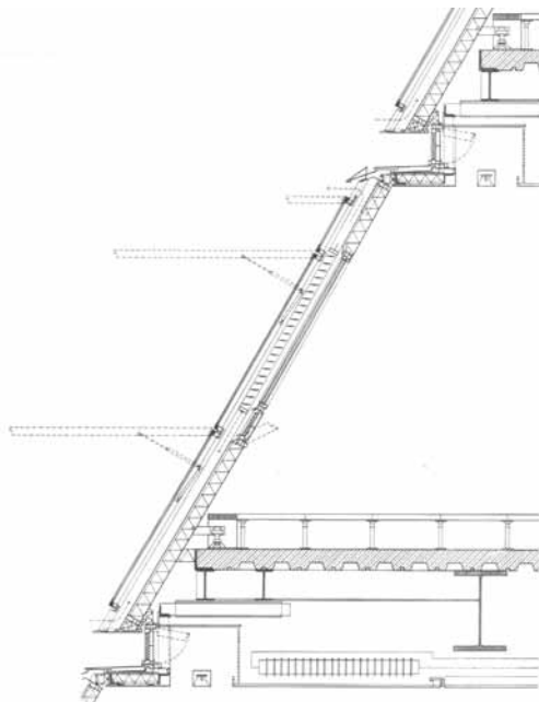
25. Installazione integrata (intercapedine vetrocamera): tipologia a lamelle.
