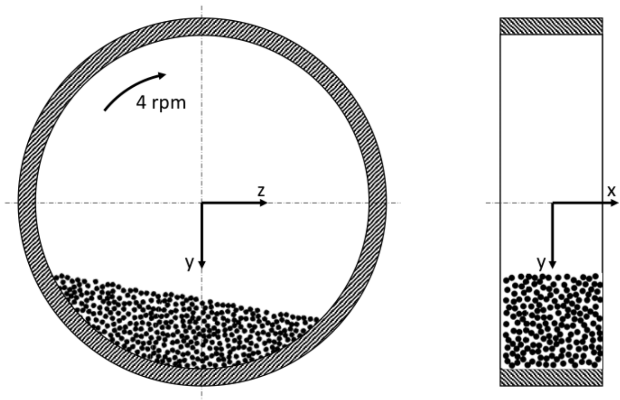
Fig. 2. DEM domain.
