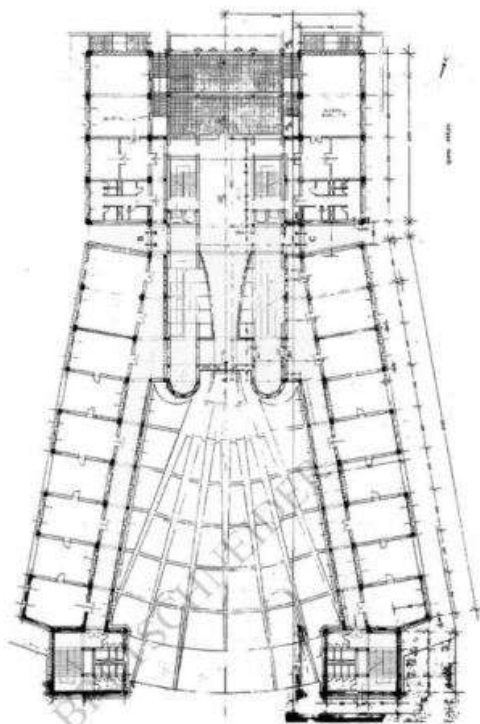
Fig. 4 - Claudia D'Amato Guerrieri, Facoltà di Agraria, Reggio Calabria, 1986/1993. Pianta del piano terreno. Claudia D'Amato Guerrieri, Faculty of Agriculture, Reggio Calabria, 1986/1993. Ground floor plan.
