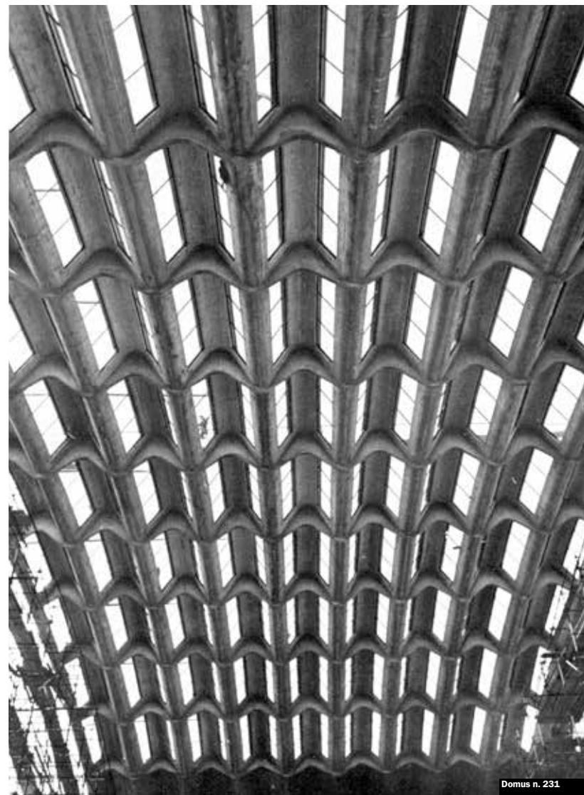
1948 È di Pier Luigi Nervi la volta con elementi prefabbricati del Salone dell'auto a Torino/ Pier Luigi Nervi used prefabricated elements for the vault of the Turin Motor Show
