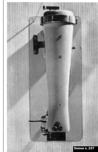
1949 Gio Ponti disegna la macchina da cucire Visetta per la Visa di Voghera/ The Visetta sewing machine by Gio Ponti for the Visa company in Voghera, Lombardy
