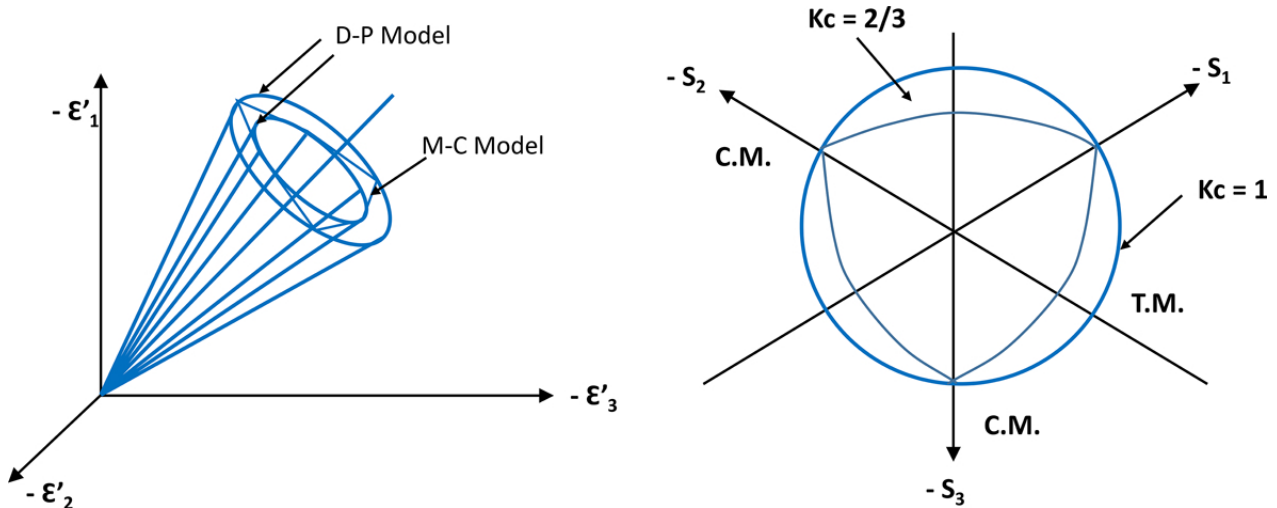
Fig. (3). ABAQUS modified Drucker-Prager strength domain.
