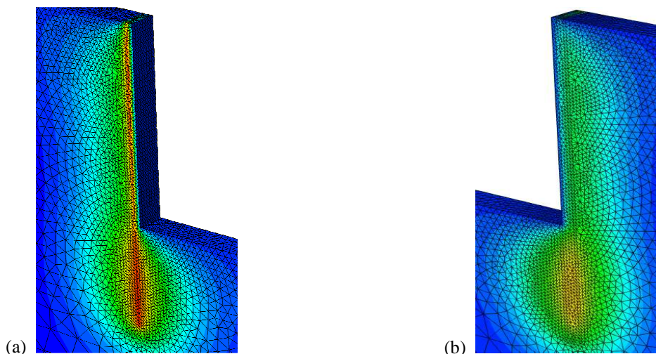
Fig 4. Campo di incremento di temperatura \Delta T(x) nei pressi del diaframma, nella condizione più gravosa, sui piani: (a) x = 1.2 m, e (b) x = 0 .m ( \Delta T min÷max = 0÷11.5 °C).
