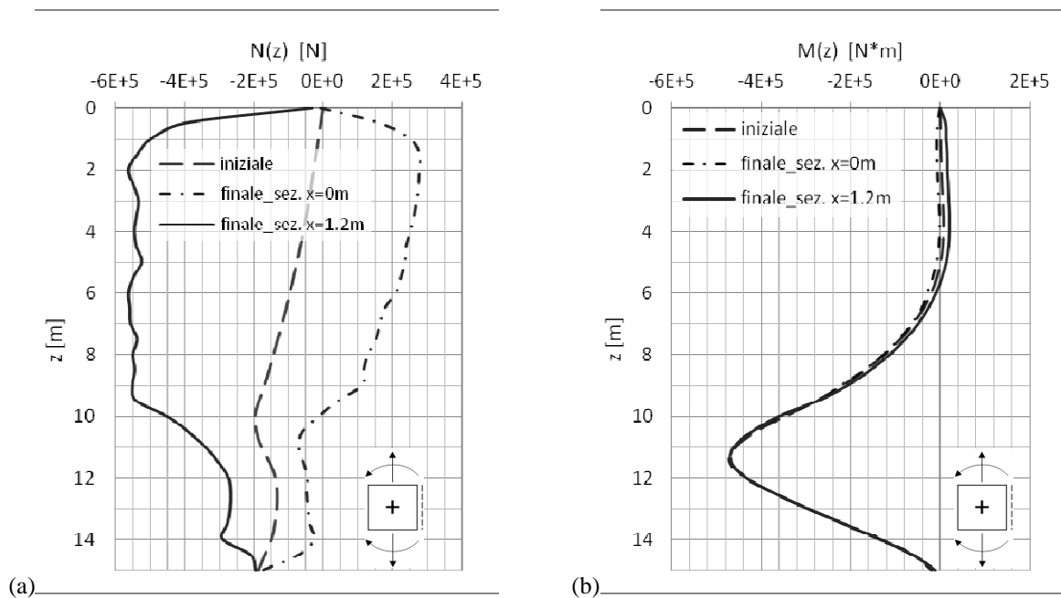
Fig 5. Diagrammi di azione assiale (a) e momento flettente (b) del diaframma, nei piani x = 1.2\text{ m} e x = 0\text{ m} .
