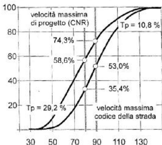
Distribuzione percentile delle velocità e percentuale di veicoli con V > V^*
