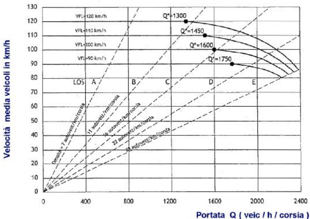
Curve velocità - portata per autostrade e strade assimilabili
