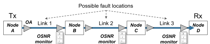
Fig. 1. NICT’s Sendai testbed setup
