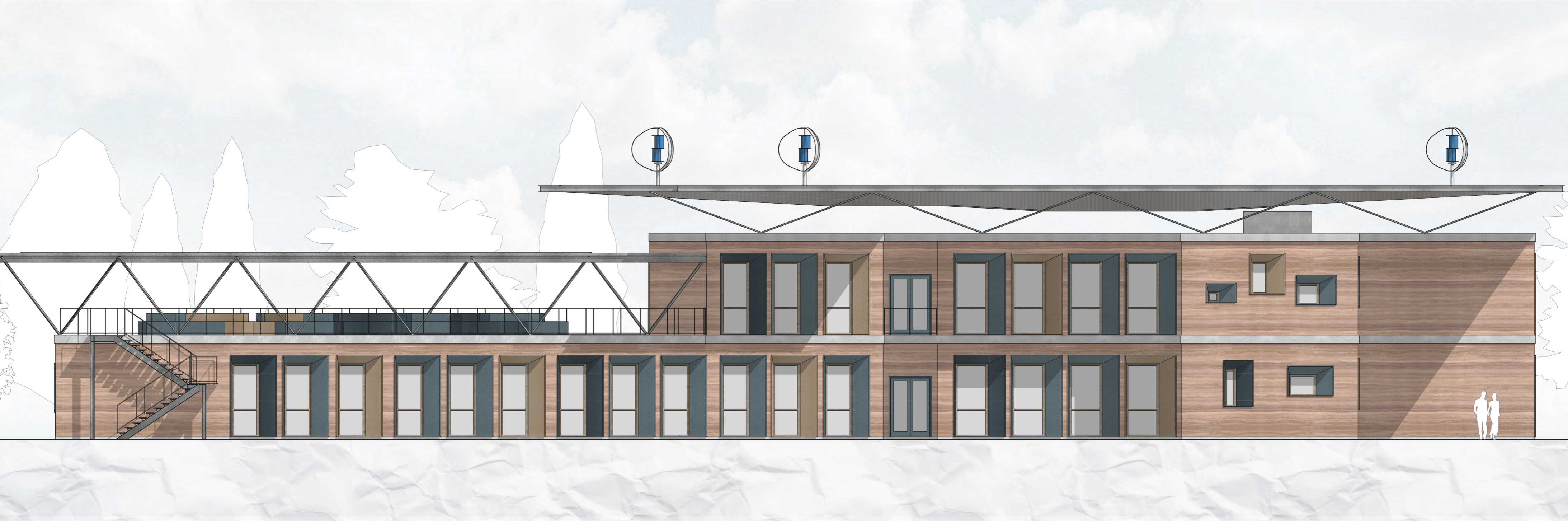
LICEO SCIENTIFICO G. GALILEI, SPADAFORA (ME) - PROSPETTO NORD, SCALA 1:100
