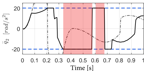
(d) Joint 2 acceleration
