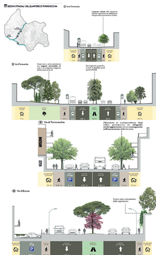
Fig. 11 - Principali sezioni stradali del Quartiere Torrevecchia / Main street sections of the District Torrevecchia (Source: Elaboration by RU Sapienza Università di Roma).
