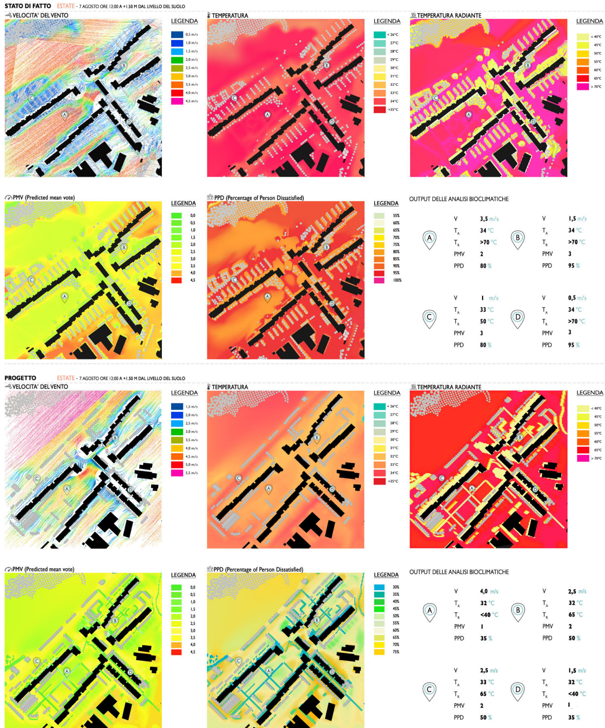
Fig. 44 - Schemi concept di progetto e simulazione dei comportamenti termo e fluidodinamici nei valori estremi d'estate nello stato di ante operam e post operam / Design and simulation of thermal and fluid-dynamic behaviors in summer extreme values in the ante operam and post operam state (Source: Elaboration by Research Unit Sapienza Università di Roma).
