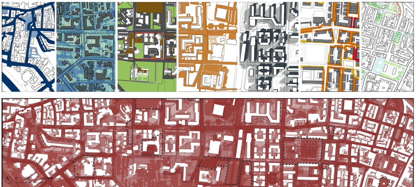
Fig. 21- Transetto di riqualificazione. In alto in sequenza le mappe tematiche degli indicatori di criticità, in basso la mappa delle aree prioritarie di intervento / Renovation transect . Above: the sequence of the thematic maps of the critical indicators; below: the map of the priority areas of intervention (Source: Authors' elaboration).
