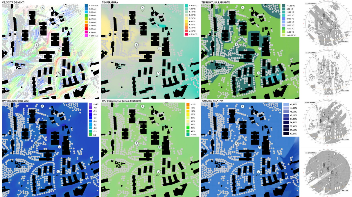
Fig. 52 - Simulazione dei comportamenti ambientali termo e fluidodinamici oltre che il soleggiamento nei valori estremi d'estate e d'inverno nello stato ante operam del quartiere di Pineto-Valle Aurelia / Simulation of the environmental thermo and fluid dynamic behaviors as well as the sunshine in the extreme summer and winter values in the ante operam state of the Pineto-Valle Aurelia district (Source: Elaboration by Research Unit Sapienza Università di Roma).
