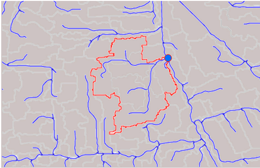
Fig. 18 - Esempio di raggruppamento delle aree colanti con un unico punto di arrivo / Example of drainage micro-areas grouping with a single arrival point (Source: Authors' elaboration).
