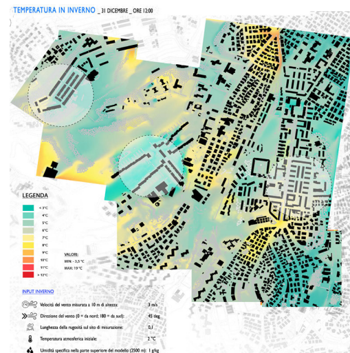
Fig. 22 - Temperature in inverno dell'area oggetto di sperimentazione / Temperature in Winter of the area under experimentation (Source: Elaboration by Research Unit Sapienza Università di Roma).
