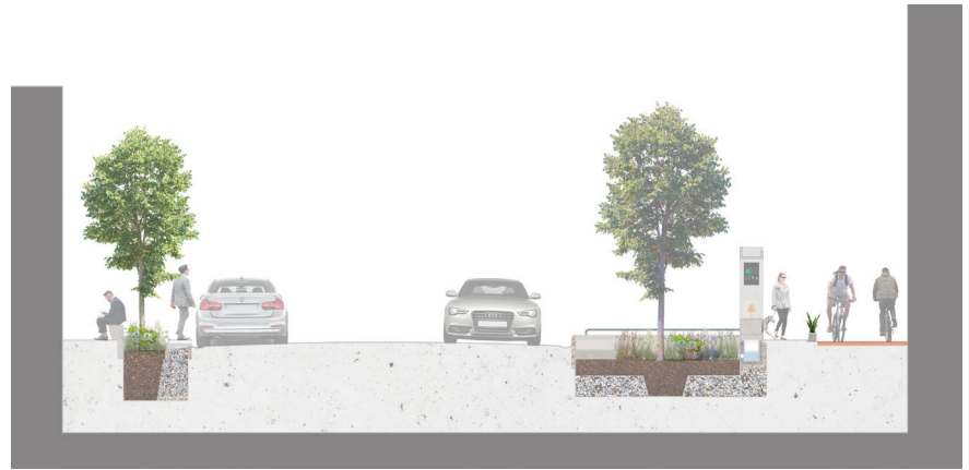
Fig. 49 - Sezione trasversale tipo con GSI / Cross-section type with GSI (Source: Authors' elaboration).
