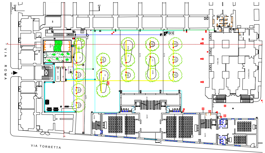
Fig. 45 - Planimetria del progetto idraulico di recupero delle acque meteoriche / Plan of the hydraulic project for the rainwater harvesting (Source: Authors' elaboration).
