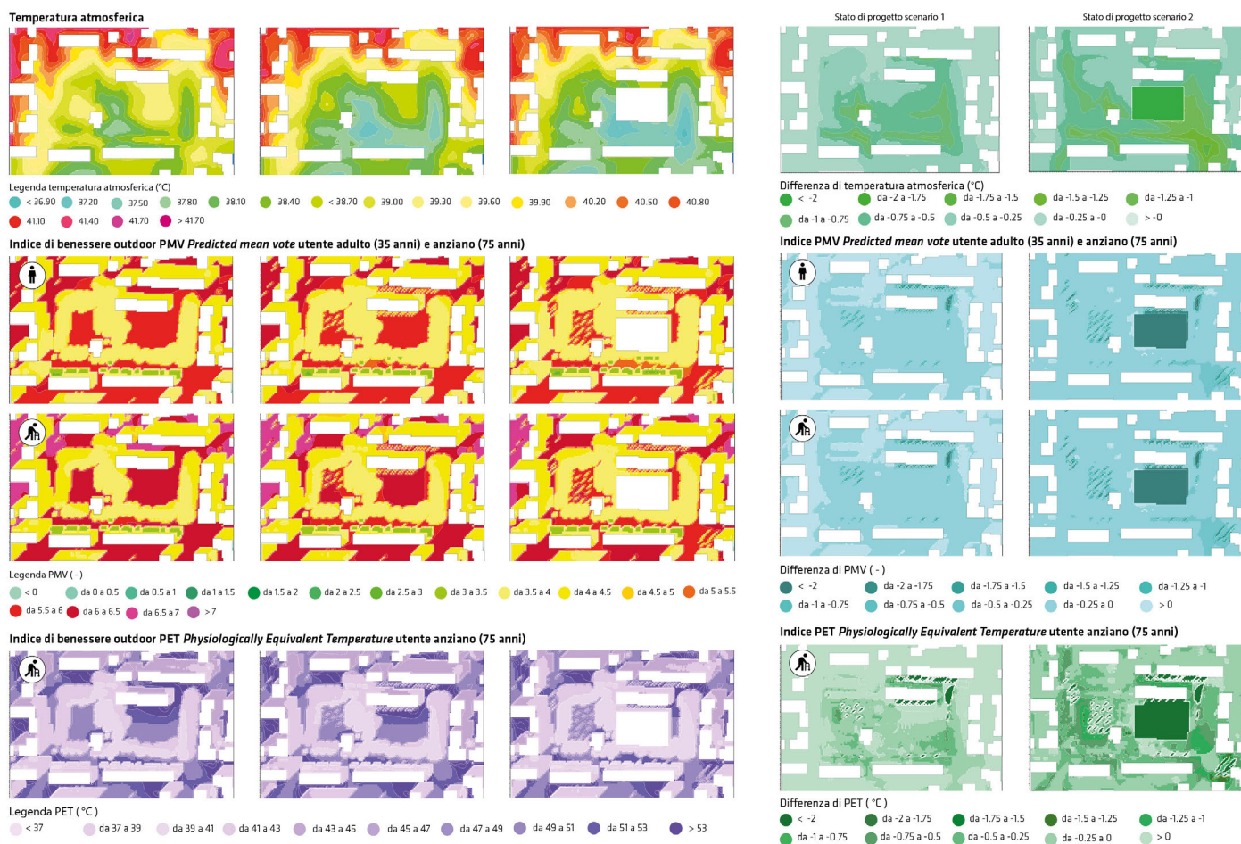
Fig. 34 - Output termici e comparazione sull'area campione di piazza Togliatti / Thermal output and comparison on the case study of Piazza Togliatti (Source: Authors' elaboration).
