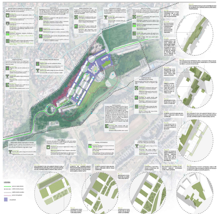
Fig. 2 - Approccio alla sperimentazione: masterplan del quartiere ERP di Quartaccio, Roma. Concept di riferimento e definizione dei sistemi progettuali e tecnologici che caratterizzano l’intervento di adaptive design / Approach to experimentation: master plan of the ERP District of Quartaccio, Rome. Concept of reference and definition of the design and technological systems that characterize the adaptive design intervention (Source: Elaboration by Research Unit Sapienza Università di Roma).
