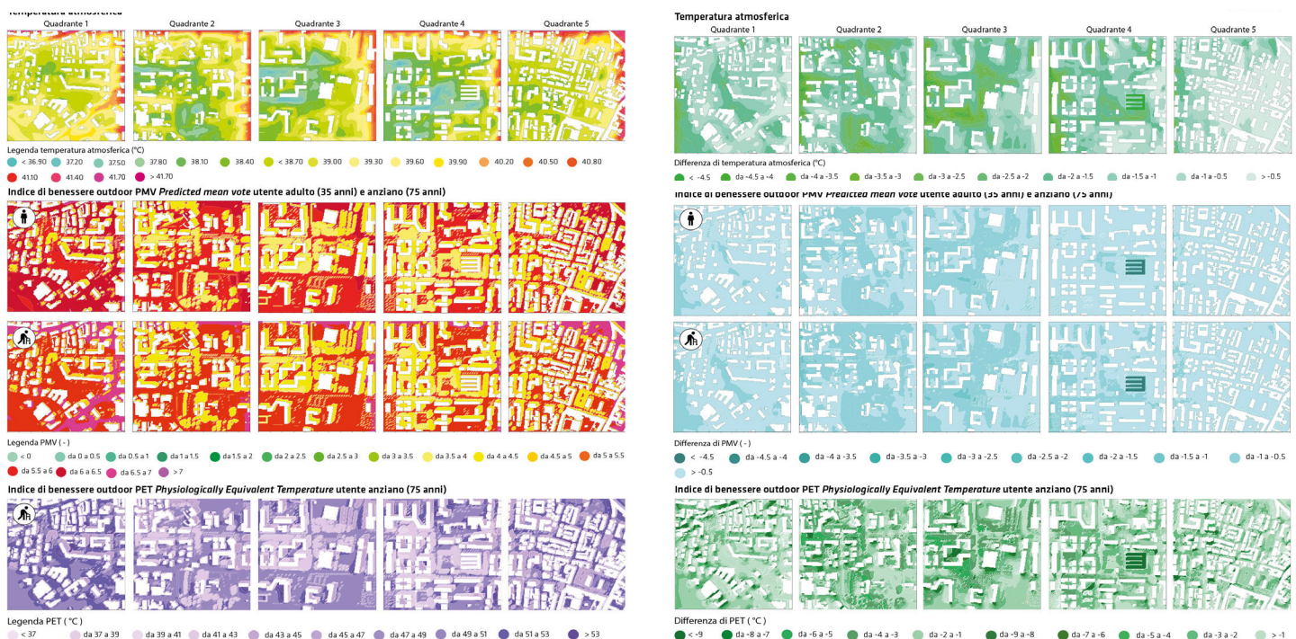
Fig. 27 - Estrapolazioni ex post e comparazioni ENVI-met di temperature atmosferiche e indici di benessere PMV e PET sul transetto di riqualificazione / Ex post ENVI-met extrapolations and comparison of the atmospheric temperatures and PMV and PET indices on the renovation transect (Source: Authors' elaboration).
