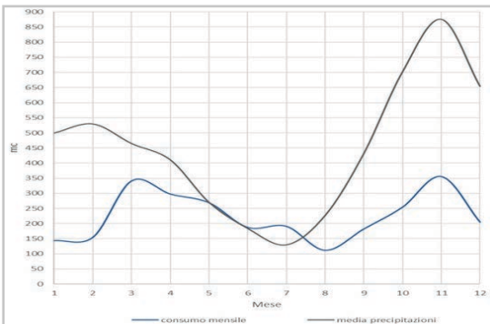
Fig. 46 - Sovrapposizione su base mensile delle curve di volume d'acqua stoccabile e consumato / Overlapping of stored and consumed water volume curves on monthly basis (Source: Authors' elaboration).
