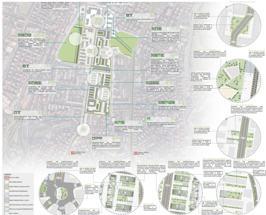
Fig. 26 - Masterplan del quartiere ex IACP di Primavalle, Strategie, Misure di intervento e Azioni di retrofitting degli spazi pubblici / Master plan of the former IACP District of Primavalle, strategies, intervention measures and retrofitting of public spaces (Source: Elaboration by Research Unit Sapienza Università di Roma).
