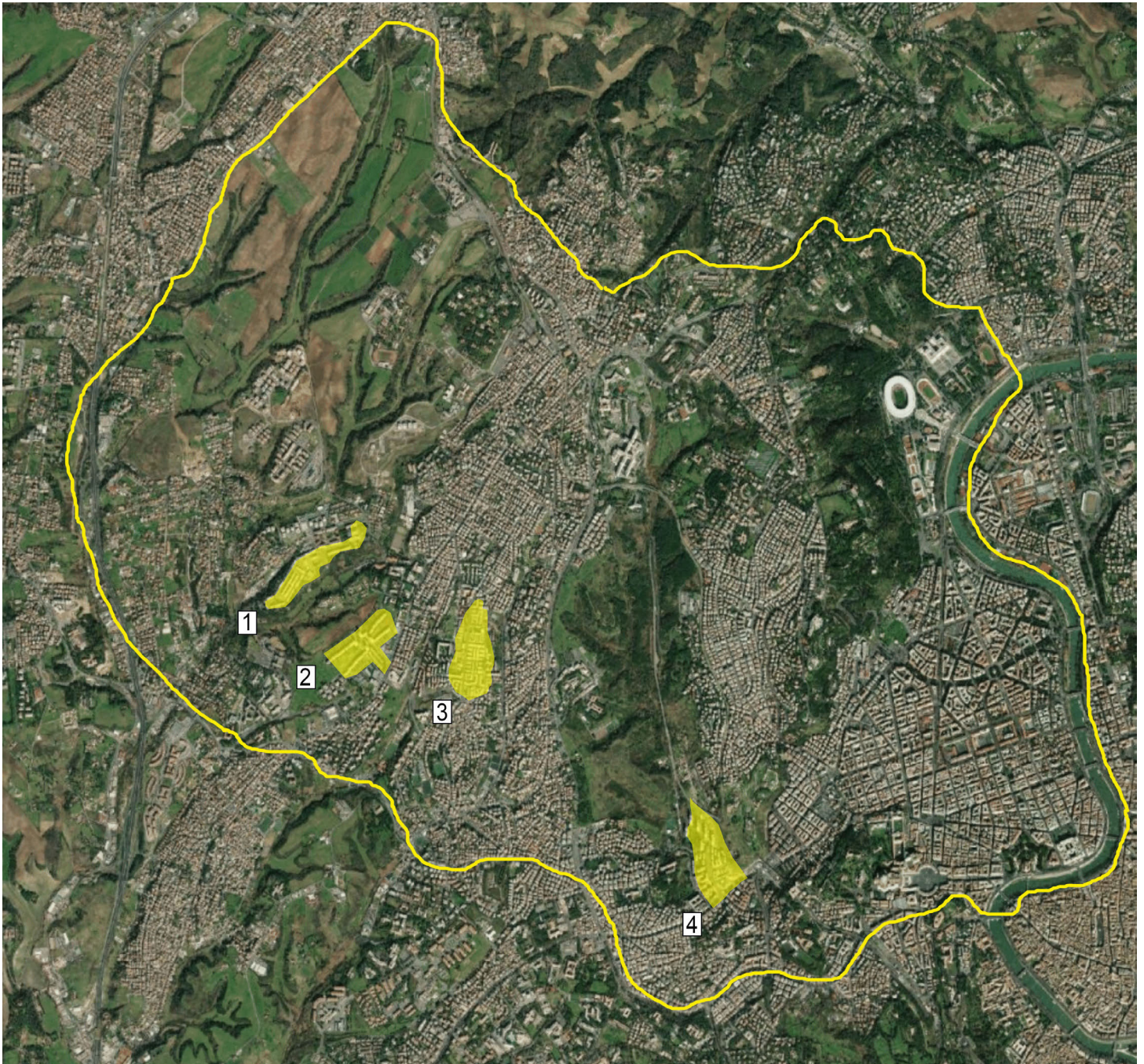
Roma, Zona Nord-Ovest, ortofoto elaborata su Geoportale Regione Lazio. Individuazione della Macroarea urbana oggetto della sperimentazione, e delle 4 aree ove si sono sviluppati i progetti dimostratori: 1. Quartaccio; 2. Torvecchia; 3. Primavalle; 4. Pineto-Valle Aurelia / Rome, North-West Area, orthophoto elaborated on Geoportale Regione Lazio. Identification of the urban Macro-area object of the experimentation, and of the 4 areas where the demonstrator projects have been developed: 1. Quartaccio; 2. Torvecchia; 3. Primavalle; 4. Pineto-Valle Aurelia (Source: Elaboration by Research Unit Sapienza Università di Roma).
