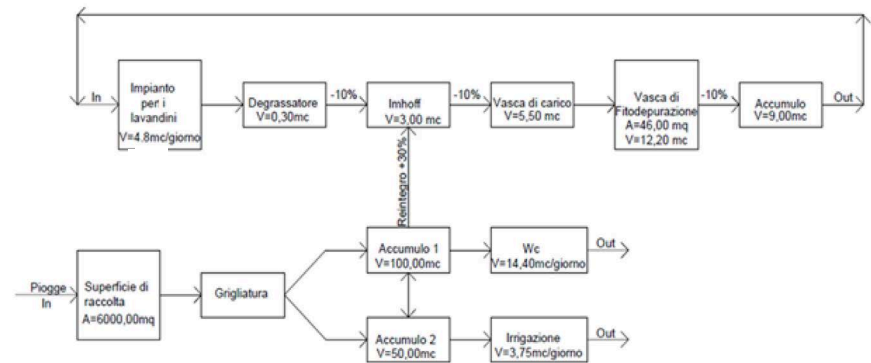
Fig. 47 - Schema di funzionamento dell'impianto di stoccaggio, fitodepurazione e riutilizzo / Operating diagram of the storage, phyto-purification and reuse plant (Source: Authors' elaboration).
