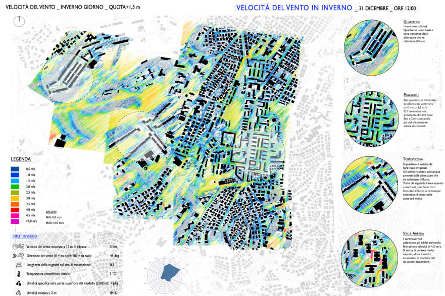
Fig. 17 - Velocità del vento ( Wind Speed ) in inverno dell'area oggetto di sperimentazione / Wind Speed in Winter of the area under experimentation (Source: Elaboration by Research Unit Sapienza Università di Roma).
