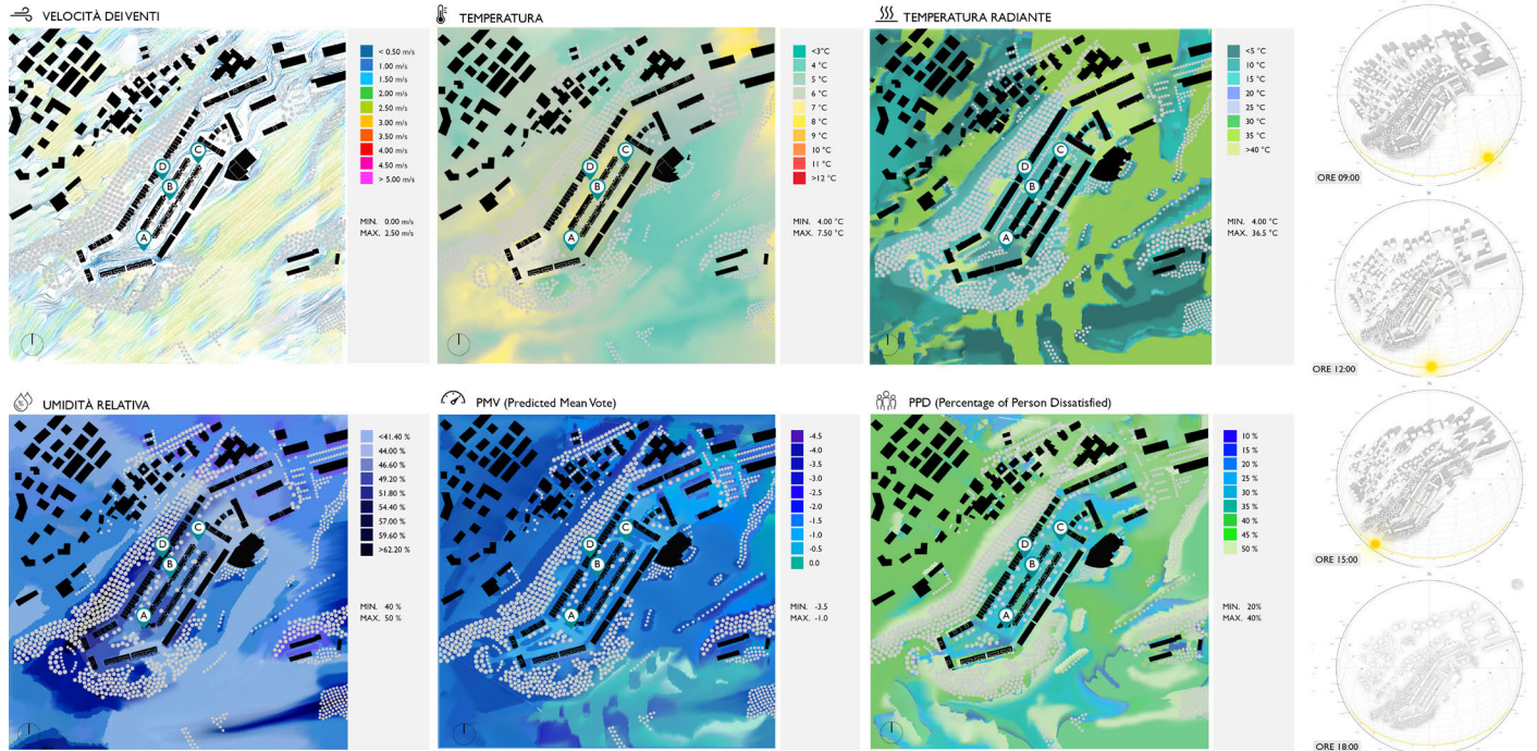
Fig. 51 - Simulazione dei comportamenti ambientali termo e fluidodinamici oltre che il soleggiamento nei valori estremi invernali con confronto ante operam e post operam del quartiere di Quartaccio / Simulation of the thermo and fluidodynamic environmental behaviors as well as the sunshine in the extreme winter values with ante operam and post operam comparison of the Quartaccio district (Source: Elaboration by Research Unit Sapienza Università di Roma).
