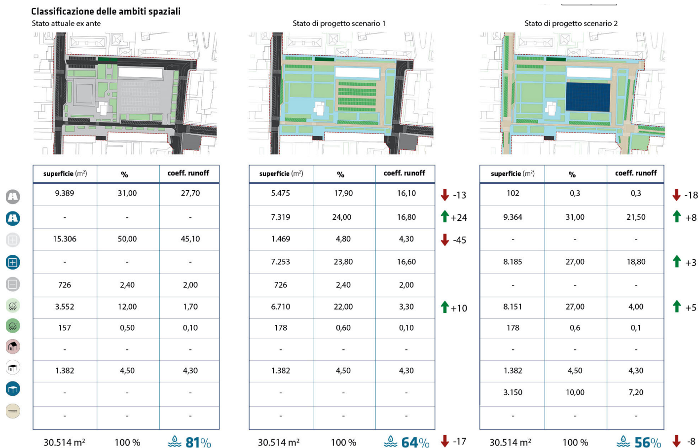
Fig. 35 - Applicazione del metodo predittivo sull'area campione di Piazza Togliatti: stato attuale e scenari metaprogettuali / Application of the predictive method on the case study of Piazza Togliatti: the existing situation and the two designed scenarios (Source: Authors' elaboration).
