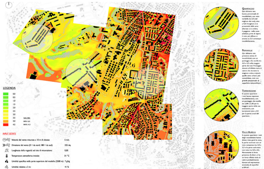
Fig. 20 - PMV ( Predicted Mean Vote ) in estate dell'area oggetto di sperimentazione / PMV (Predicted Mean Vote) in Summer of the area under experimentation (Source: Elaboration by Research Unit Sapienza Università di Roma).
