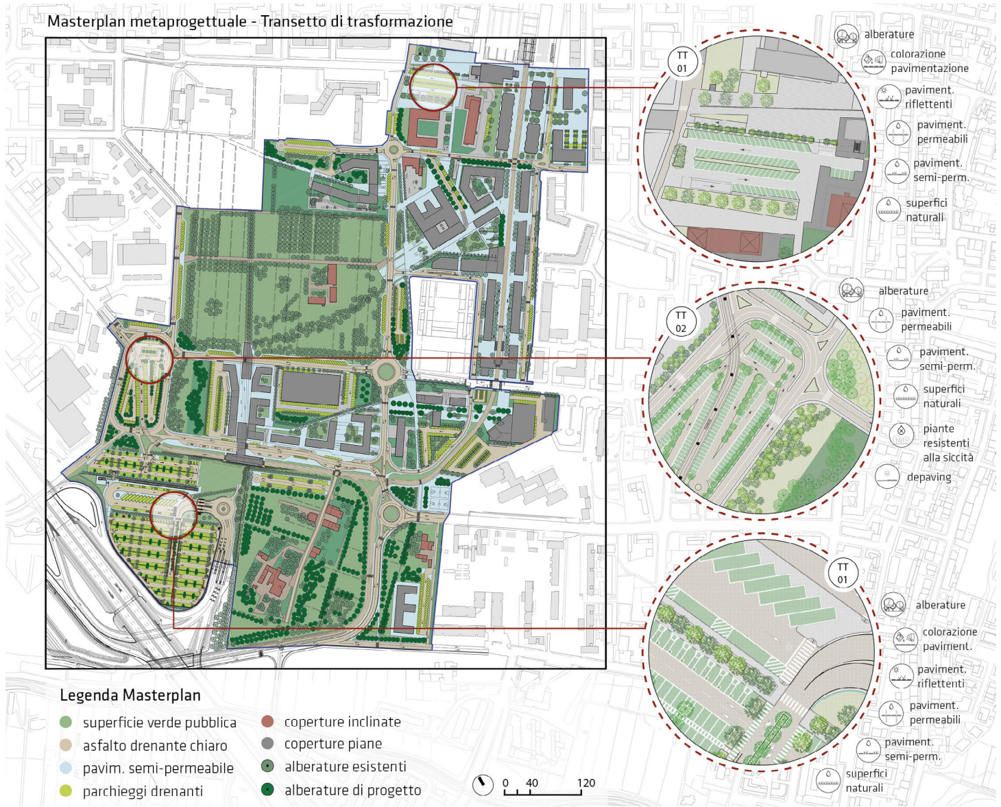
Fig. 26 - Soluzioni tecnologiche e spaziali adottate nella spina del transetto di trasformazione/ Technological and spatial solutions adopted in the intervention area of the development transect (Source: Authors' elaboration).
