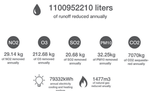
Fig. 28 - Quantificazione dei benefici ambientali del masterplan ottimizzato / Quantification of the optimized master plan environmental benefits (Source: Elaboration by Nora Oquendo).
