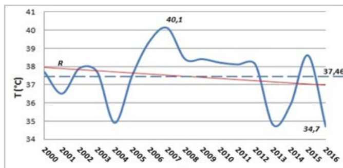
Fig. 5 - Diagramma dell'escursione termica annua E_{ta} (°C) calcolata dai dati registrati dalla stazione di Grazzanise / Diagram of the annual temperature range E_{ta} (°C) calculated from temperature data recorded by the Grazzanise station.
