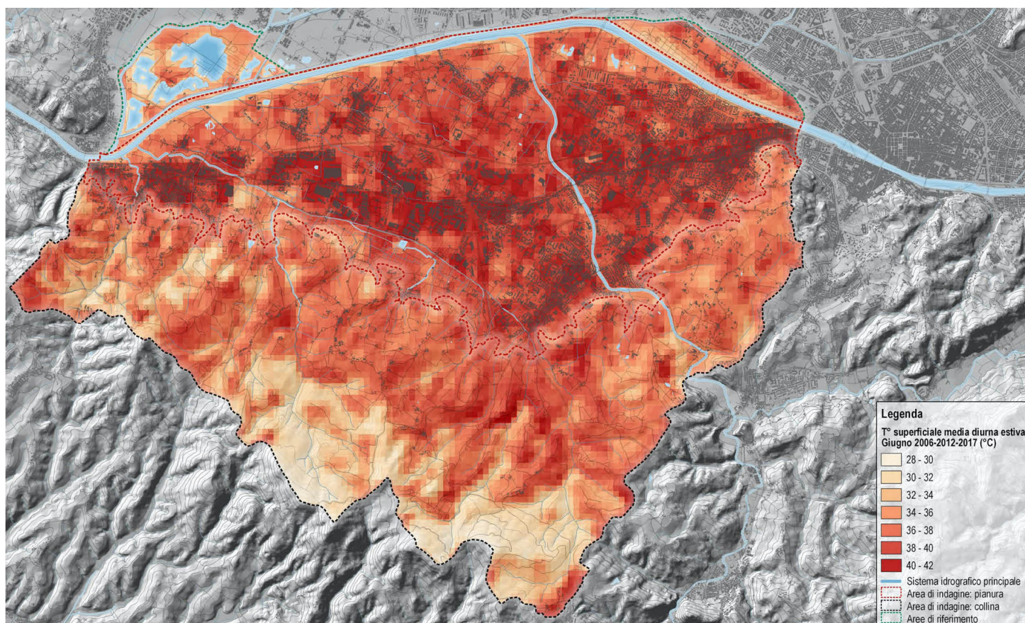
Fig. 3 - Analisi relative alle temperature superficiali medie diurne esitive riferite al mese di Giugno 2006-2012-2017 / Analysis of the average summer surface temperature referred to the months of June 2006-2012-2017 (Source: Elaboration by Giulia Guerri).
