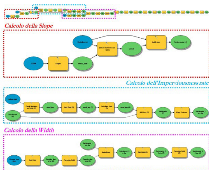
Fig. 18 - Abstract grafico del tool creato per calcolo dei dati relativi ai sottobacini di drenaggio urbano necessari per la simulazione idraulica / Graphical Abstract of the automated tool to calculate the input data of each sub-catchment for hydraulic simulation (Source: Authors' elaboration).
