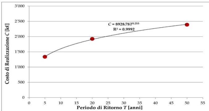
Fig. 22 - Andamento del costo di costruzione ottimale per T = 5, 20 e 50 anni./ Construction costs-return period correlation for T = 5, 20 and 50 years (Source: Authors' elaboration).
