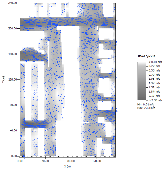
Fig. 42 - Modellizzazioni della velocità del vento nelle aree campione con software ENVI-met / ENVI-met software wind speed models in the pilot areas (Source: Authors' elaboration).
