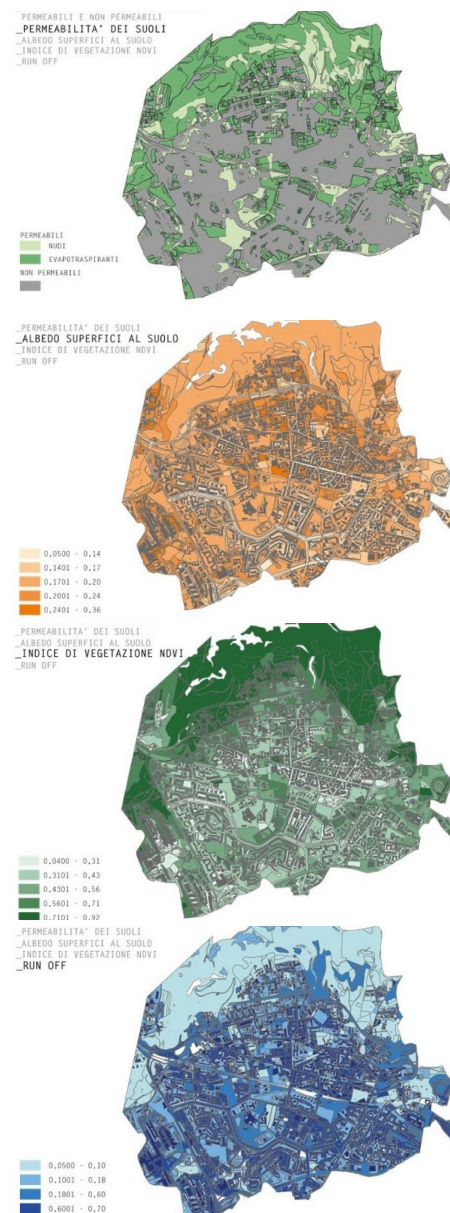
Fig. 8 - Carte tematiche riferite ai valori assunti da 4 indicatori che offrono una descrizione indiretta dei livelli di vulnerabilità alle heavy rains e alla heat wave : permeabilità dei suoli, albedo delle superfici al suolo, indici NDVI e di runoff / Thematic maps referring to the values assumed by 4 indicators that offer a description of the levels of vulnerability to heavy rains and heat wave: soil permeability, albedo of soil surfaces, NDVI and runoff indexes (Source: Elaboration by Denise Di Mauro and Sara De Rogatis, 2019).
