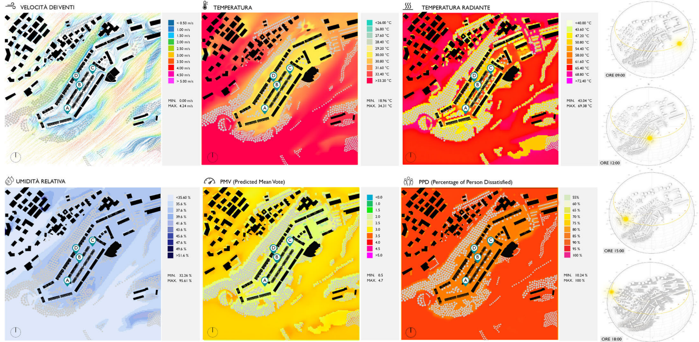
Fig. 50 - Simulazione dei comportamenti ambientali termo e fluidodinamici oltre che il soleggiamento nei valori estremi d'estate con confronto ante operam e post operam del quartiere di Quartaccio / Simulation of the thermal and fluid dynamic environmental behaviors as well as the sunshine in the extreme summer values with ante operam and post operam comparison of the Quartaccio district (Source: Elaboration by Research Unit Sapienza Università di Roma).
