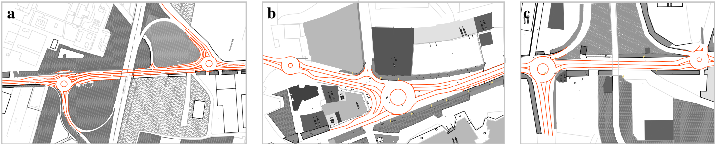
Fig. 27a, b, c - Soluzione di progetto per lo svincolo in zona ospedale (a), in zona Asse Mediano (b) e alle Colonne di Giugliano (c) / Project solution for the junction in the hospital area (a), in the Asse Mediano area (b) and at the Giugliano Columns (c) (Source: Authors' elaboration).
