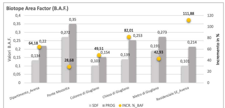
Fig. 39 - Variazioni degli indicatori specifici delle aree campione / Specific indicators variations in the sample areas (Source: Authors' elaboration).
