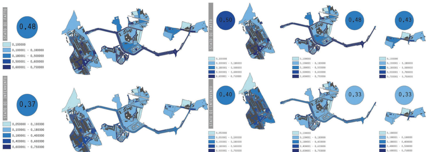
Fig. 31 - Confronto del runoff allo stato di fatto e post-intervento, alla scala di masterplan e di comparto/ Comparison of the runoff before and after design at master plan and focus scale (Source: Elaboration by Denise Di Mauro & Sara De Rogatis, 2019, Master's Degree thesis "Infrastrutture verdi per distretti climate proof. Il caso di Soccavo", supervisor Prof. Mario Losasso).
