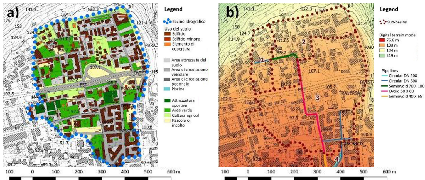
Fig. 16 - a) Database topografico classificato per usi prevalenti del suolo con indicazione del perimetro del bacino idrografico oggetto di analisi; b) Sovrapposizione di sottobacini e rete di drenaggio urbano, con indicazione delle dimensioni degli spechi, al modello digitale del terreno / a) Geographic database categorized by land uses; b) Sub-catchments borders and drainage network, categorized by pipelines typology, overlaid with digital terrain model (Source: Authors' elaboration).
