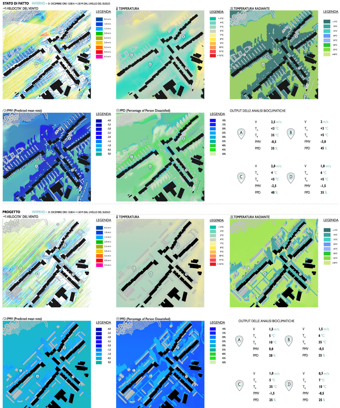
Fig. 45 - Schemi concept di progetto e emulazione dei comportamenti termo e fluidodinamici nei valori estremi d'inverno, nello stato di ante operam e post operam / Concept design schemes and emulation of thermal and fluid dynamic behaviors in extreme winter values, in ante operam and post operam state (Source: Elaboration by Research Unit Sapienza Università di Roma).
