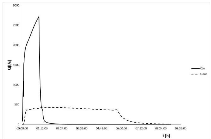
Fig. 24 - Andamento delle portate in ingresso e in uscita dalla vasca di laminazione per T = 50 anni / Flowing rate and outlet flow rate from the stormwater tank for return period T = 50 years (Source: Authors' elaboration).
