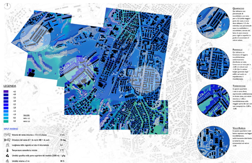
Fig. 21 - PMV ( Predicted Mean Vote ) in inverno dell'area oggetto di sperimentazione / PMV (Predicted Mean Vote) in Winter of the area under experimentation (Source: Elaboration by Research Unit Sapienza Università di Roma).
