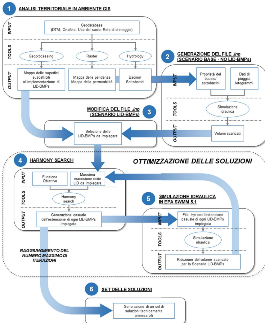
Fig. 14 - Flowchart per il dimensionamento e la localizzazione ottimale di superfici LID-BMPs / Flowchart for LID-BMPs optimal sizing and localization (Source: Authors' elaboration).
