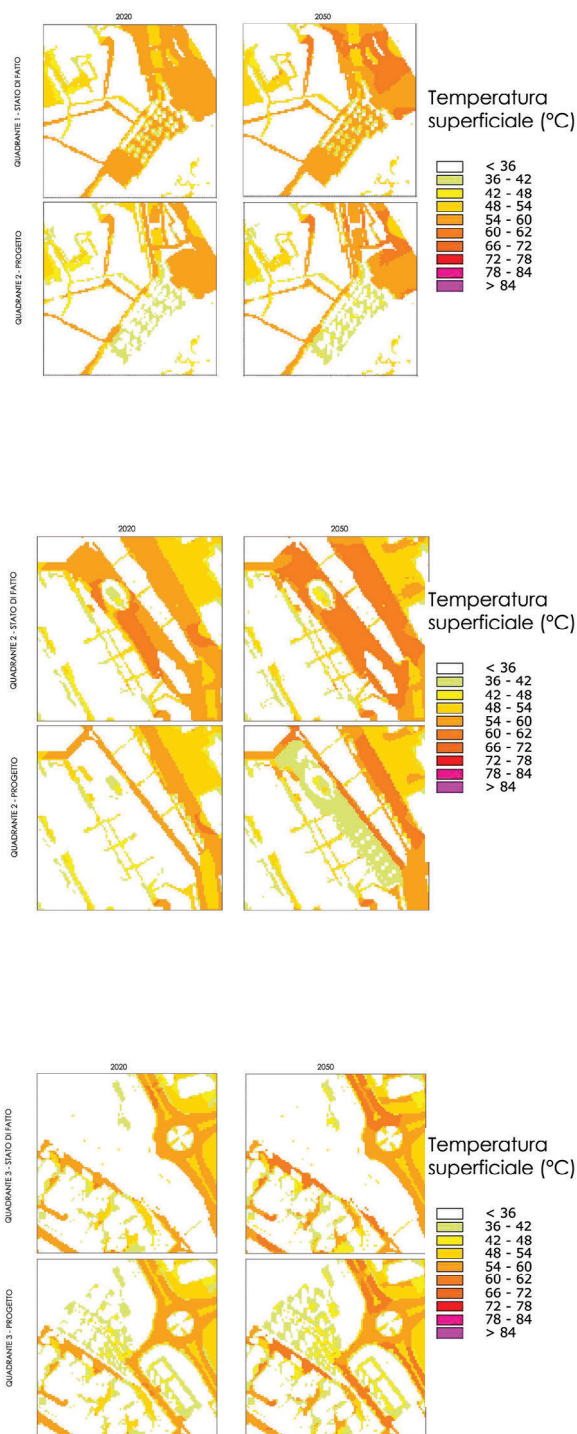
Fig. 32 - Riqualficazione degli spazi aperti a Monte Sant'Angelo. Verifica della temperatura superficiale tramite simulazioni Envi-MET / Upgrading of open spaces in Monte Sant'Angelo. Surface temperature by Envi-MET simulations (Source: Elaboration by Michele Lambiase, 2020).
