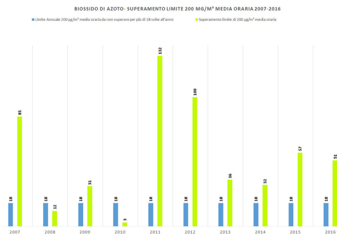
Fig. 10 - Superamento dei valori soglia di Biossido di Azoto ( NO_2 ) su base annua nell'ultimo decennio / Exceeding of the threshold values of Nitrogen Dioxide ( NO_2 ) on an annual basis in the last decade (Source: ARPA Lombardia weather station data processing closer to the Sub-area).
