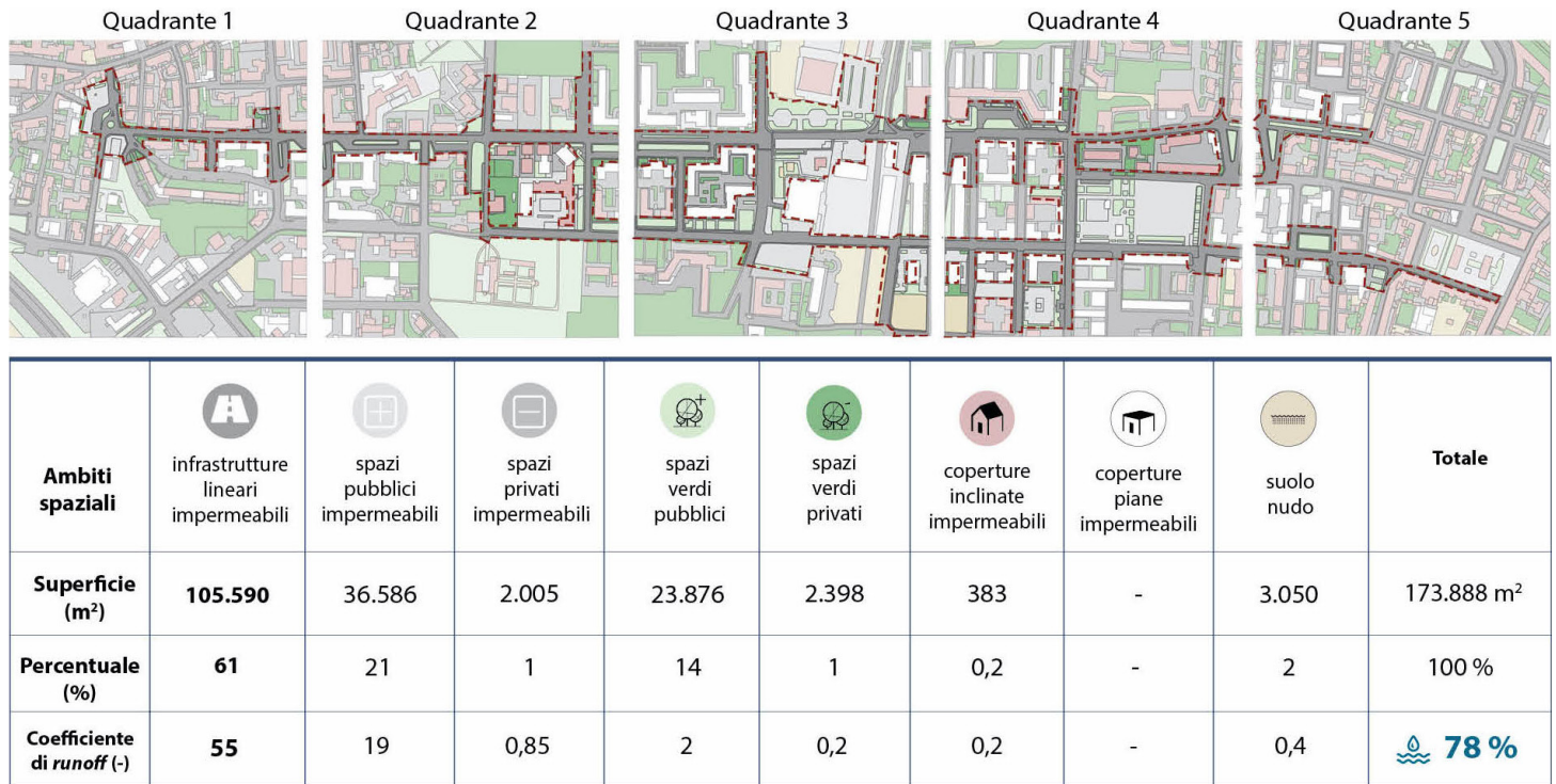
Fig. 18 - Planimetria del transetto di riqualificazione con riportati gli ambiti spaziali individuati e i rispettivi valori superficiali, percentuali e indice di runoff / Plan of the renovation transect showing the spaces identified and the respective spaces, percentage and runoff values (Source: Authors' elaboration).
