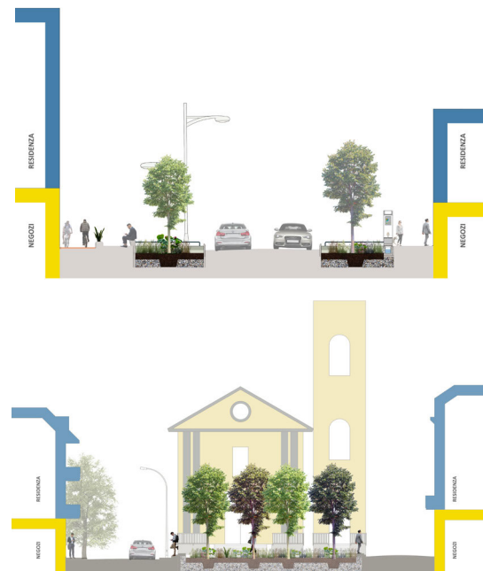
Fig. 32 - Sezioni di progetto per le aree campione a Giugliano / Project sections for sample areas in Giugliano (Source: Authors' elaboration).
