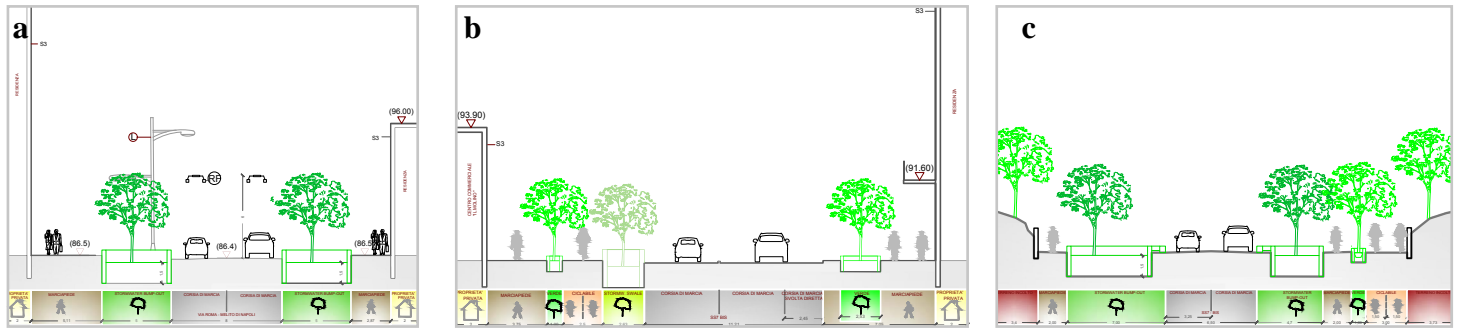
Fig. 26a, b, c - Sezioni stradali tipo di progetto / Road sections project type (Source: Authors' elaboration).
