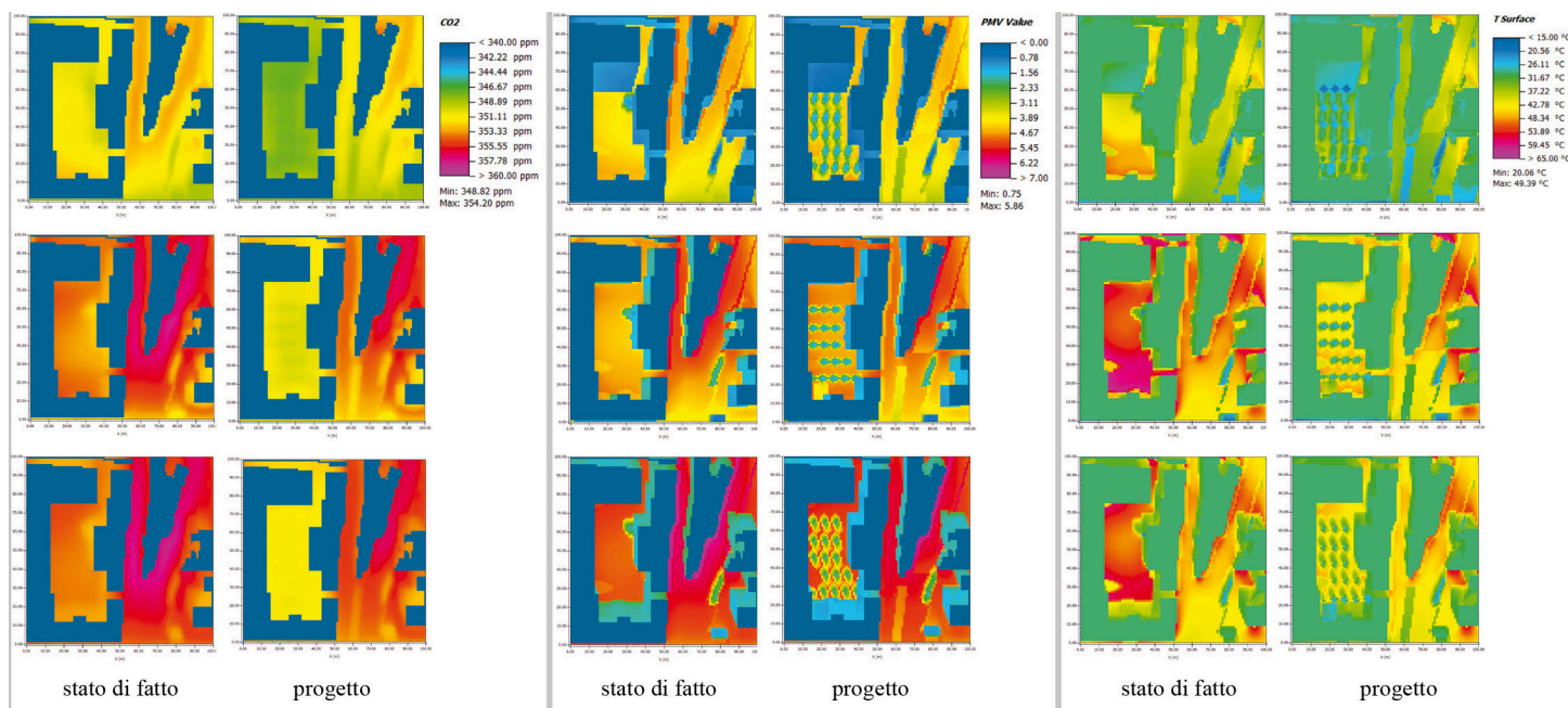
Fig. 40 - Modellizzazioni del cortile dell'Annunziata con software ENVI-met / Modelling of the Annunziata courtyard with ENVI-met software (Source: elaboration by P. Ferrara & S. Giacobbe ).
