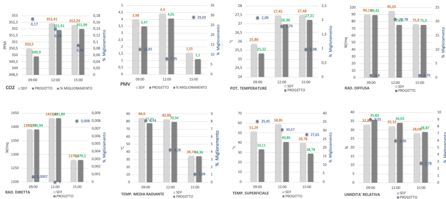
Fig. 41 - Area campione Aversa Annunziata: risultati della modellazione mediante software ENVI-met./ Aversa Annunziata pilot area: ENVI-met modeling results (Source: Authors' elaboration).
