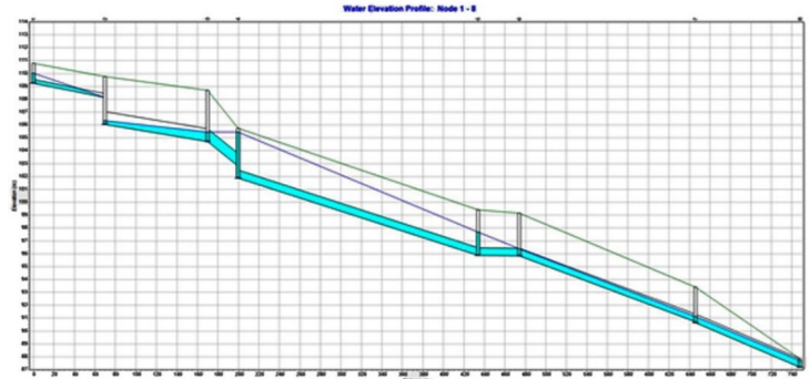
Fig. 21 - Andamento del profilo di corrente nel sistema di drenaggio (per d = 1 h e T = 5 anni) per il caso (a) senza intervento (scenario base) e (b) con la soluzione LID ottimizzata / Current Profile ( d = 1 h and T = 5 years) for (a) Baseline scenario, without LID-BMPs and (b) Design scenario with optimal LID-BMP solution (Source: Authors' elaboration).
