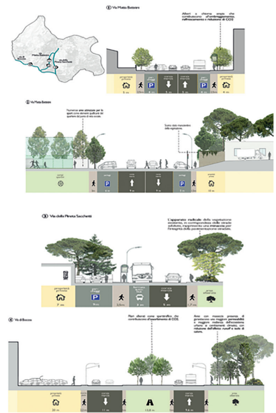
Fig. 14 - Principali sezioni stradali del Quartiere Primavalle / Main road sections of the District Primavalle (Source: Elaboration by RU Sapienza Università di Roma).
