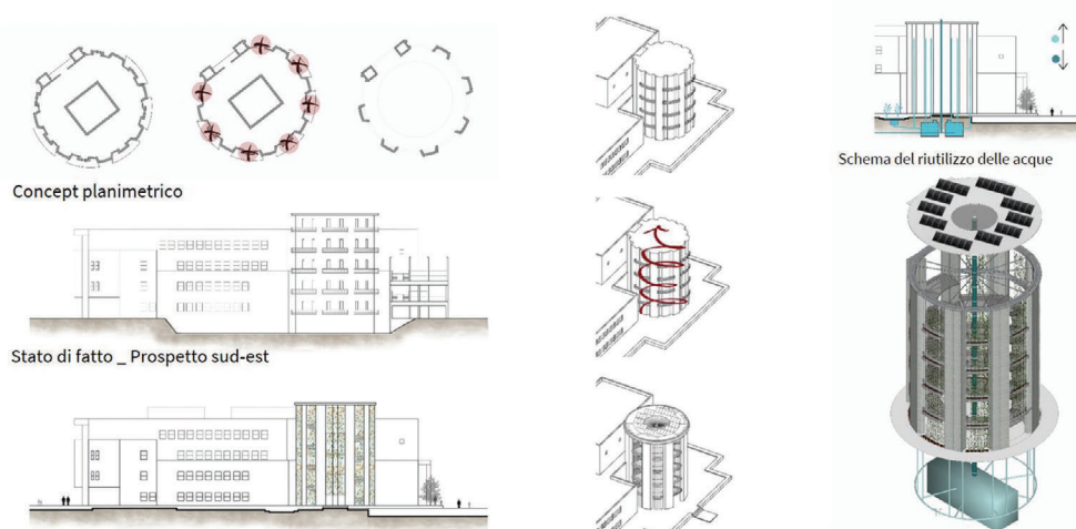
Fig. 30 - Soccavo, edificio Polifunzionale, dettaglio del blocco scala green / Soccavo, Multipurpose building, detail of the green staircase block (Source: Elaboration by Simona Cuccurese & Francesca De Luca, 2019, Master's Degree thesis "Strategie per l'adattamento ambientale e riqualificazione edilizia e urbana nel Rione Traiano. Interventi sugli spazi aperti e sull'edificio Polifunzionale", supervisor Prof. Mario Losasso).
