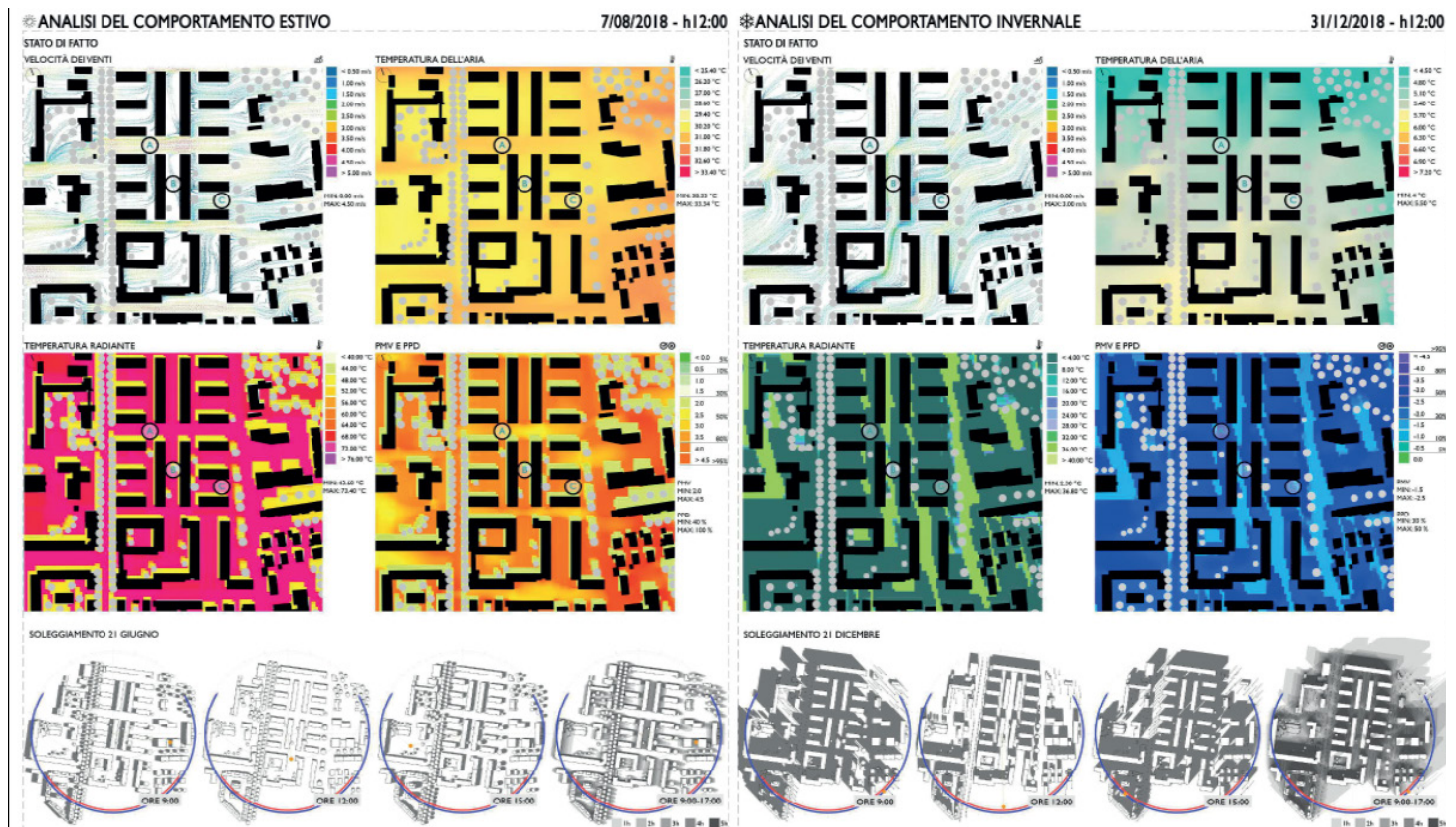
Fig. 2 - Elaborazioni di simulation and modelling relative ai principali comportamenti bioclimatici estivi e invernali nello stato ante operam e post operam dei progetti dimostratori nel quartiere ERP di Roma / Simulation and modeling processing related to the main summer and winter bioclimatic behaviors in the ex ante and ex post state of the demonstration projects in the ERP Districts of Rome (Source: Elaboration by Research Unit Sapienza Università di Roma).
