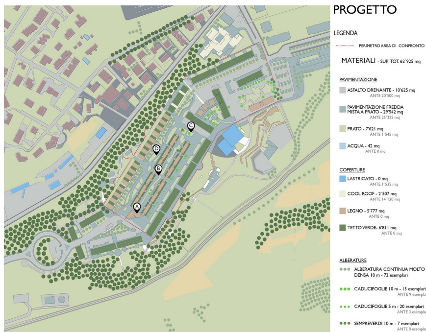
Fig. 48-49 - Planimetria dell'area di intervento di Torvecchia con indicazione delle trasformazioni del trattamento materico delle superfici ante operam (in alto) e post operam (in basso) / Planimetry of the area of intervention of Torvecchia with indication of the transformations of the material treatment of the surfaces ante operam (top) and post operam (below) (Source: Elaboration by Research Unit Sapienza Università di Roma).
