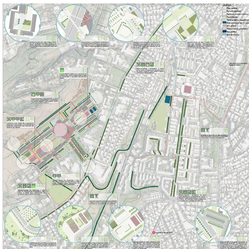
Fig. 1 - Sviluppo sperimentale nel progetto dimostratore applicato sul quartiere ERP di Primavalle, Roma, con indicazione delle strategie e misure di intervento, e delle specifiche azioni di retrofitting degli spazi pubblici / Experimental development in the demonstrator project applied to the ERP District of Primavalle, Rome, with indication of the intervention strategies and measures, and of the specific retrofitting actions of public spaces (Source: Elaboration by Research Unit Sapienza Università di Roma).
