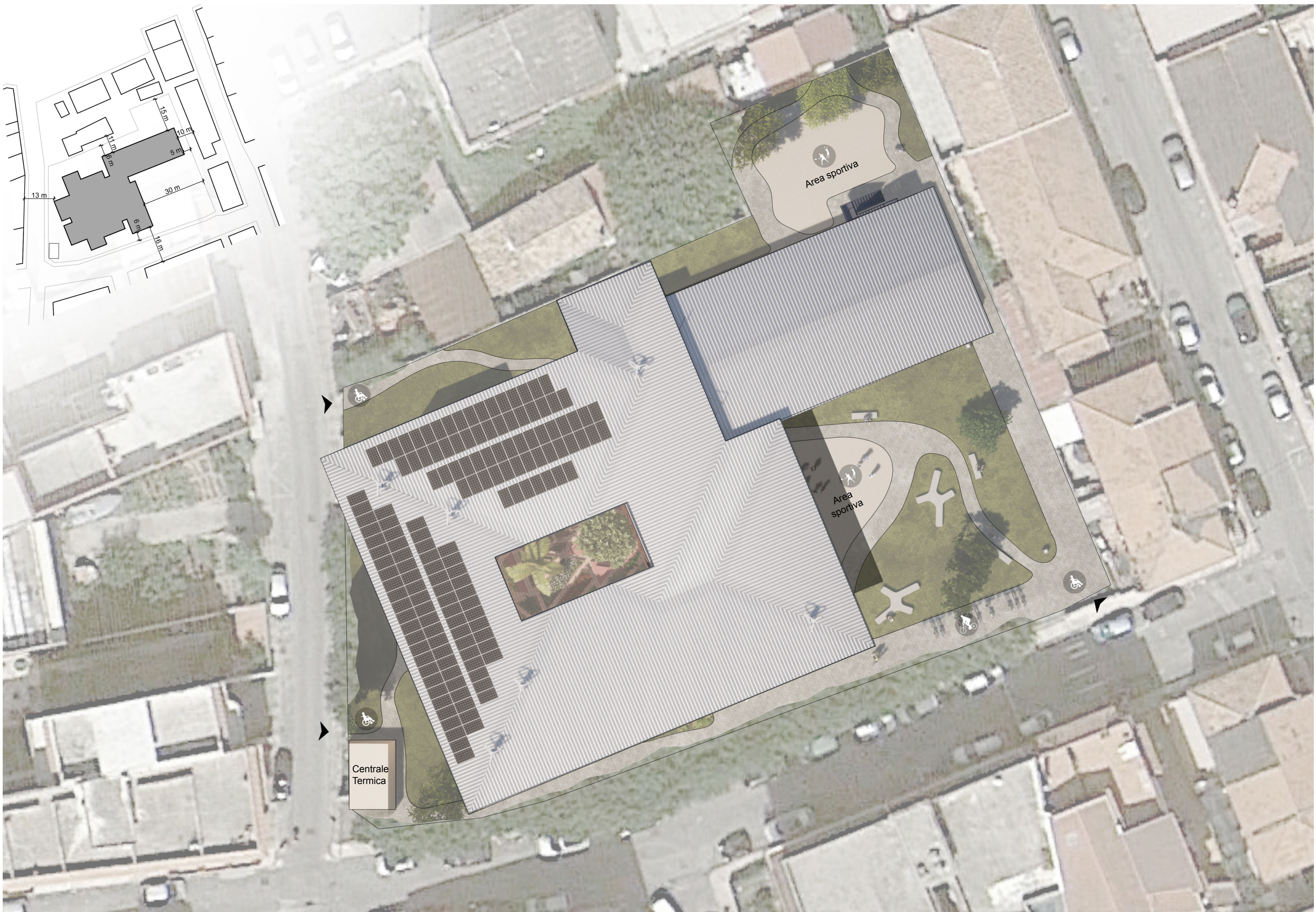
LICEO SCIENTIFICO G.GALILEI, SPADAFORA (ME) - PLANIMETRIA GENERALE, SCALA 1:200
