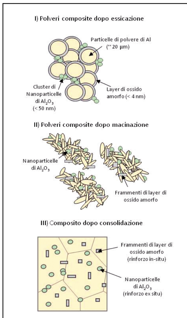
Fig. 3 - Schema dell'effetto del ball milling e del processo di consolidazione I) dopo asciugatura, le particelle di alluminio ricoperte da un ossido amorfo passivante sono rivestite da cluster di \gamma\text{-Al}_2\text{O}_3 , II) dopo la macinazione severa questi cluster e il layer di ossido passivante vengono rotti in particelle discrete, III) dopo compattazione mediante estrusione i frammenti di layer di ossido e le NP di \gamma\text{-Al}_2\text{O}_3 sono dispersi all'interno della matrice di alluminio.
