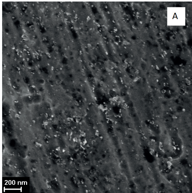
Fig. 2 - Microstruttura del MMnC (a) rinforzato con particelle generate in situ e (b) rinforzato con particelle generate in situ e aggiunte ex situ.
