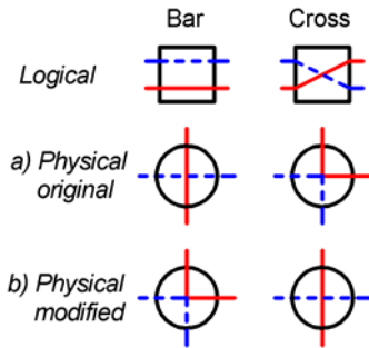
Fig. 6: Elementos de conmutación de estados lógicos vs físicos: a) correspondencia como en [20], [21]; b) nueva correspondencia física.
