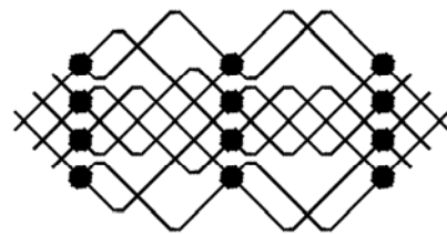
Fig. 4: Red Baseline de 8 × 8
