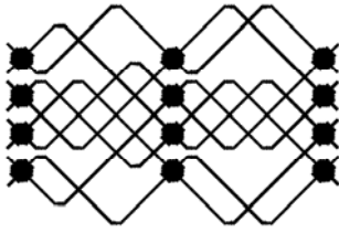
Fig. 5: Red Baseline acortada de 8 \times 8
