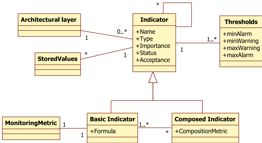
Fig. 1 Indicators meta-model
