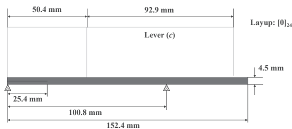
Fig. 8 MMB specimen.
