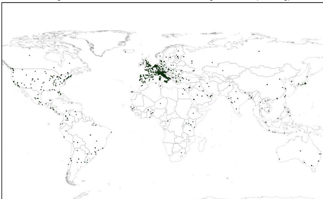
Figura 1: Fablab Torino: Localizzazione di ogni follower (lat, long)
