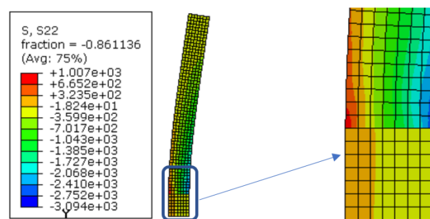
Figura 12. Sforzi verticali alla base al limite elastico (distribuzione forze lineare).
