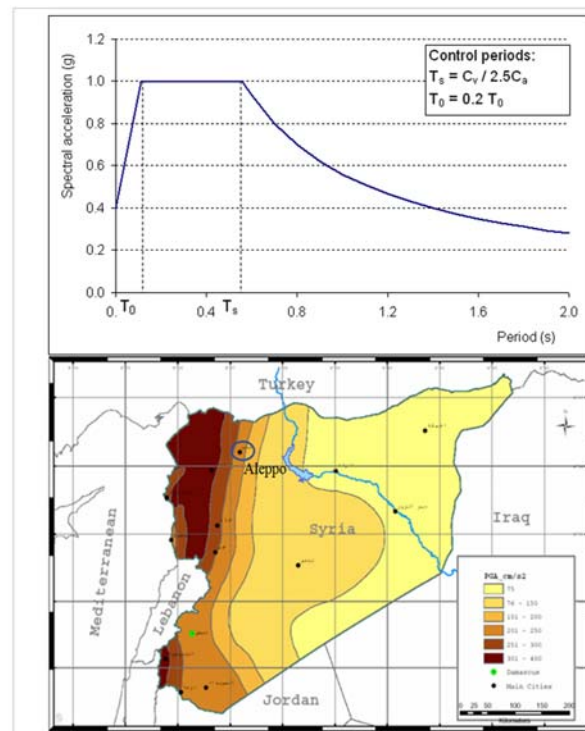
Figura 7. Mappa di pericolosità sismica e spettro di risposta previsti dalle norme siriane..
